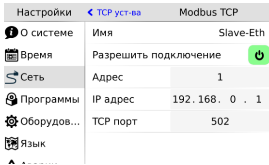
Рис. 56 – Настройка Modbus TCP slave
