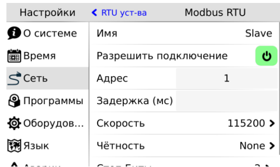
Рис. 57 – Настройка Modbus RTU slave
