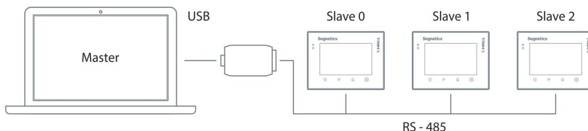
Рис. 30 – Построение сети на RS-485
