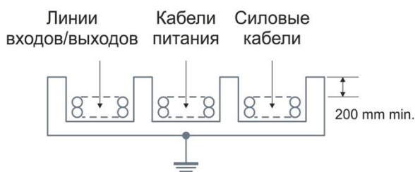
Рис. 26 - Горизонтальные каналы
